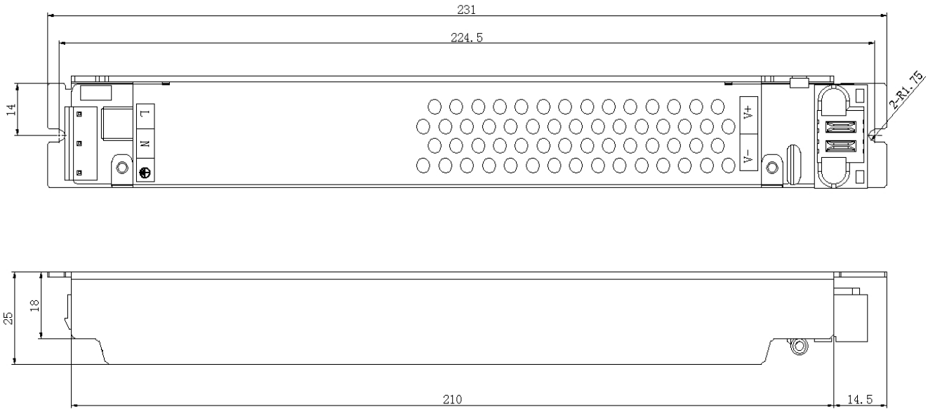
(3) CL-PAS2-200-5 (B) 外形尺寸
