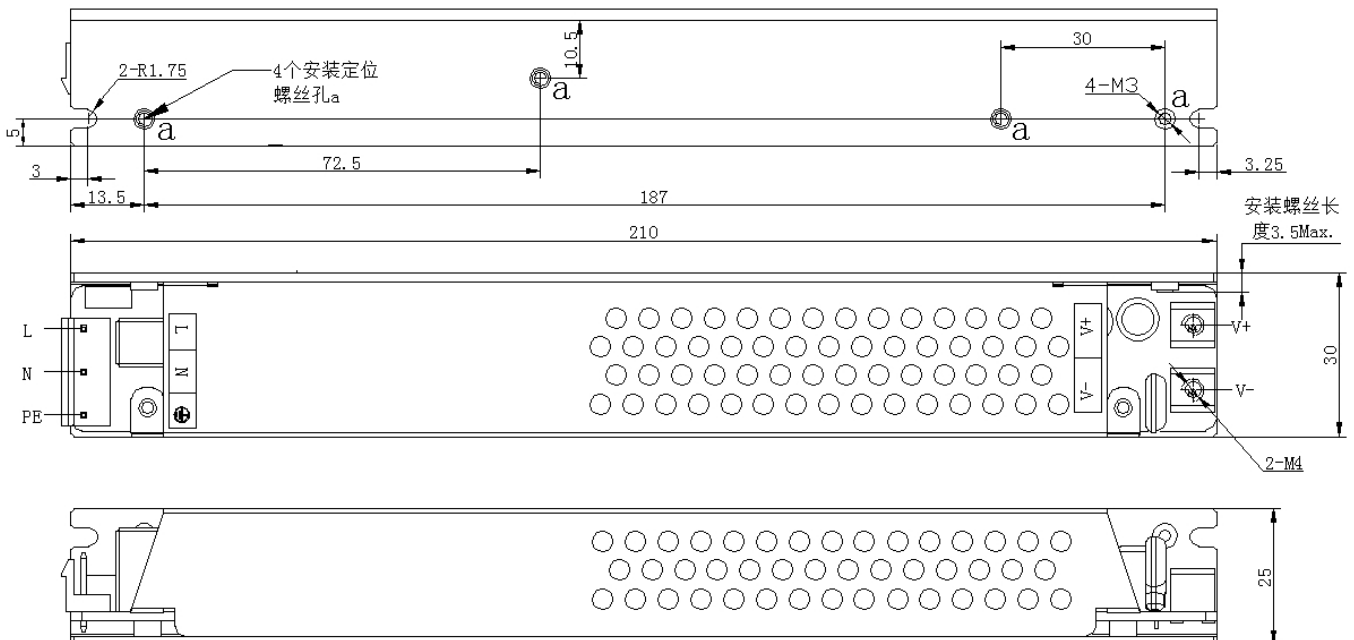
(2) CL-PAS2-200-5 (A) 外形尺寸
