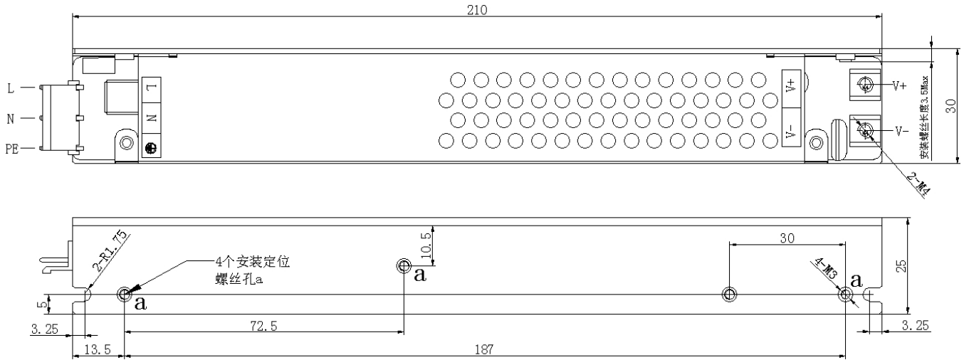
(3) CL-PAS2-200-5 (B) 外形尺寸
