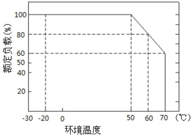
■环境温度降额曲线
